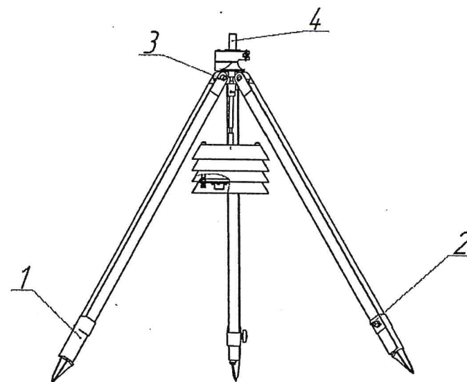
1 - тавр; 2 - зажим; 3 - барашек; 4 – опора.
